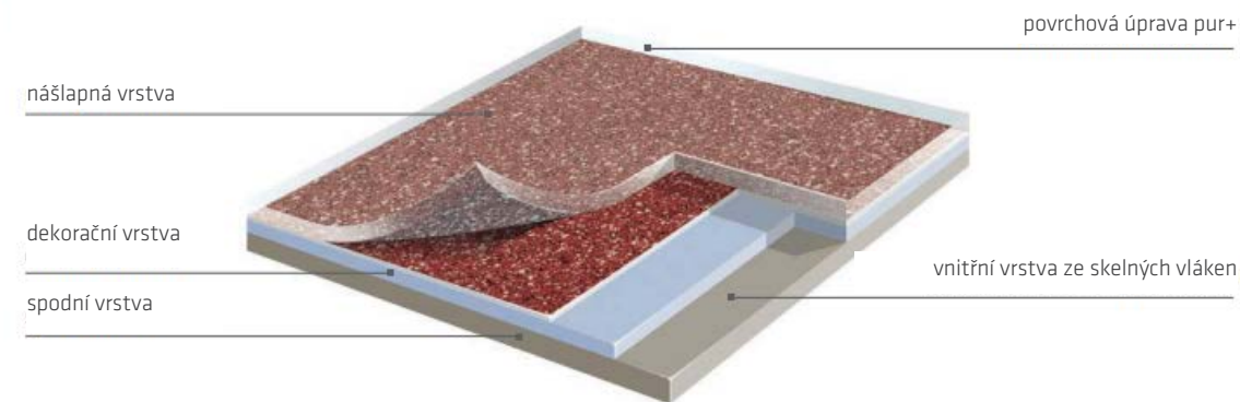
● Průřez materiálem
